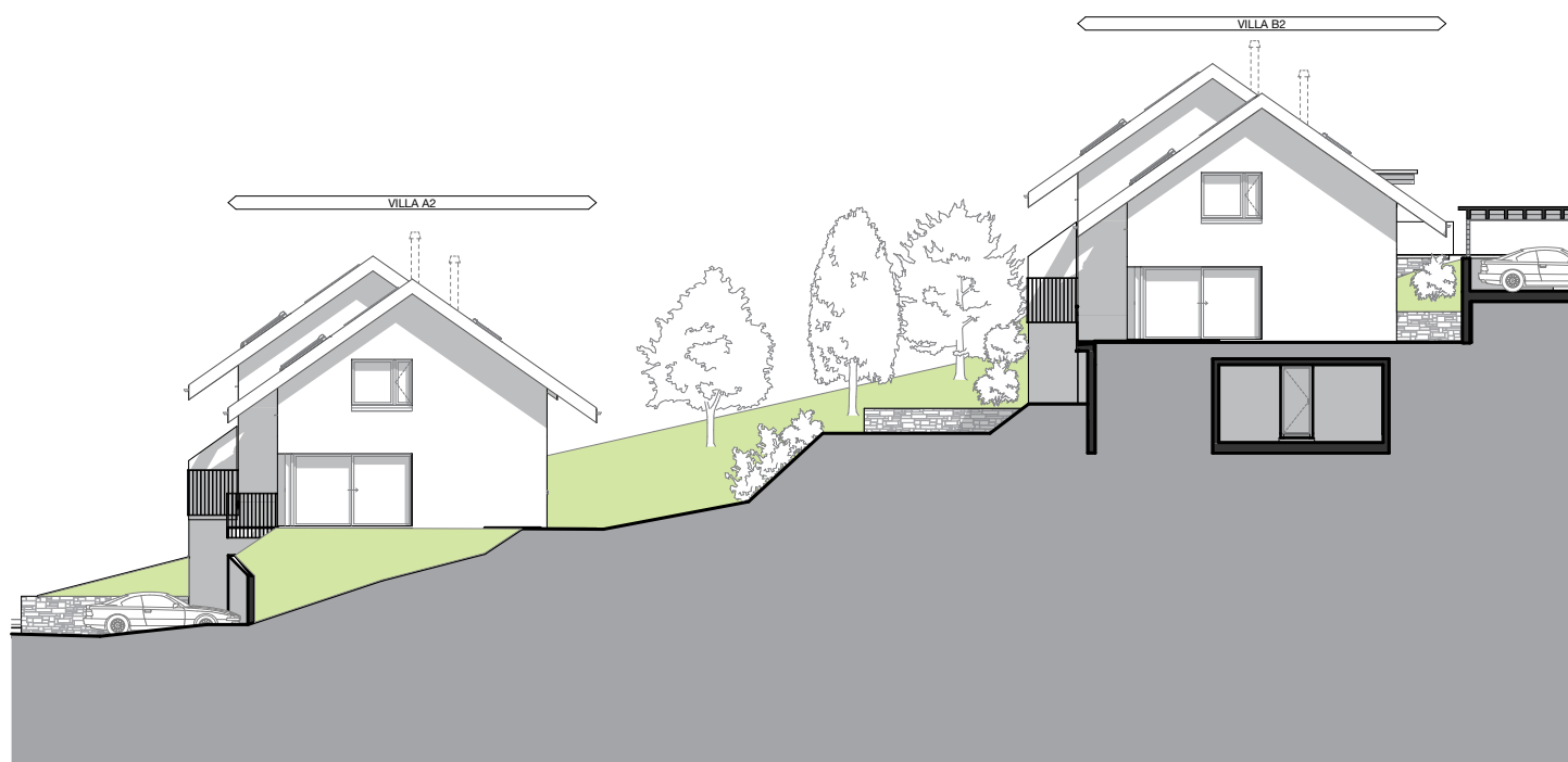
FACADE EST VILLAA2 et B2
